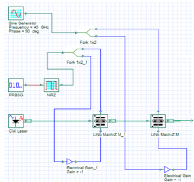
Fig. 4 Transmitter subsystem.
